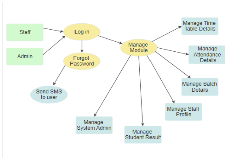
Fig. DFD level 2
