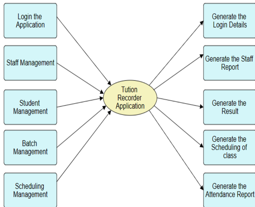
Fig. DFD level 1
